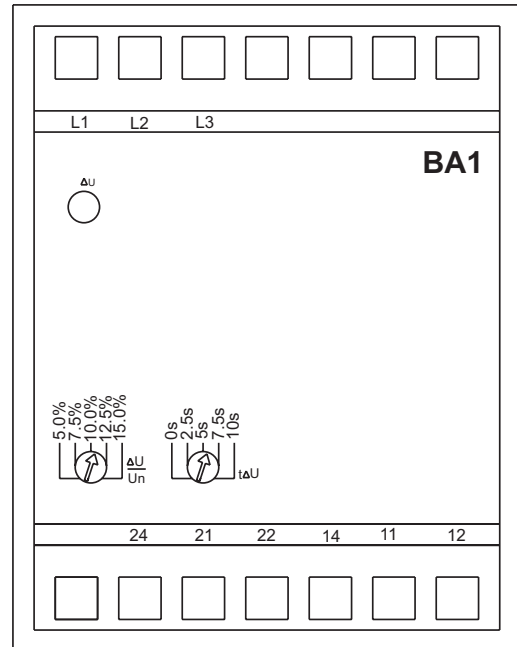
Fig. 1 : Front plate
