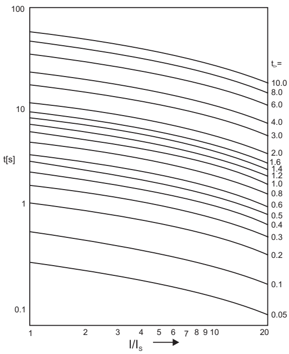
Fig. 7.6 : RXIDG-characteristic
