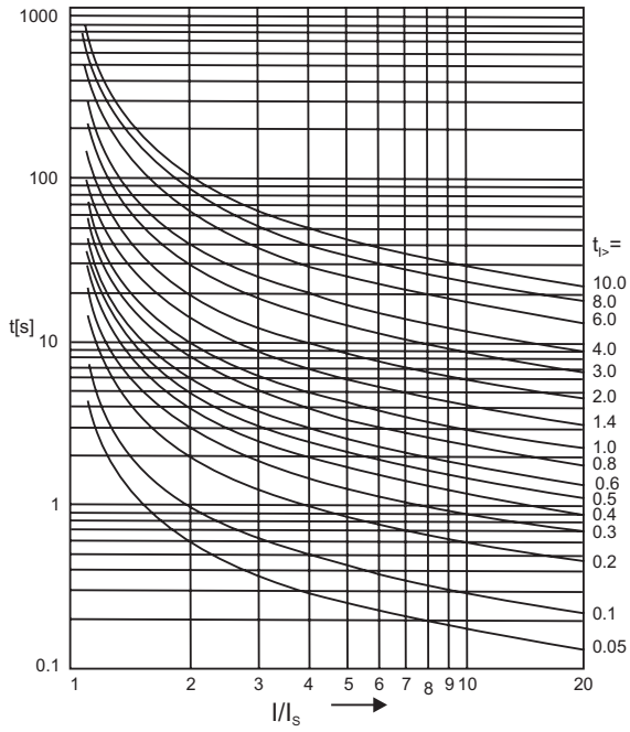
Fig. 7.1 : Normal Inverse
