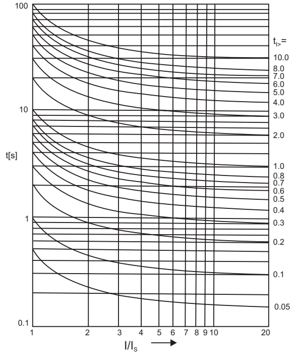
Fig. 7.4 : RI-Inverse
