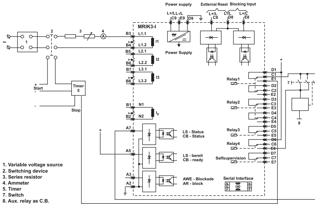
Fig. 6.1 : Test circuit
